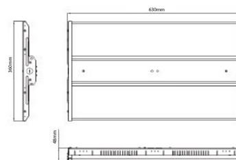
220W Dimensions
