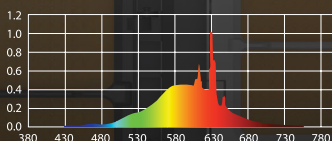
Réglage de luminaire 3000K avec optique ambre = 2200K CCT
